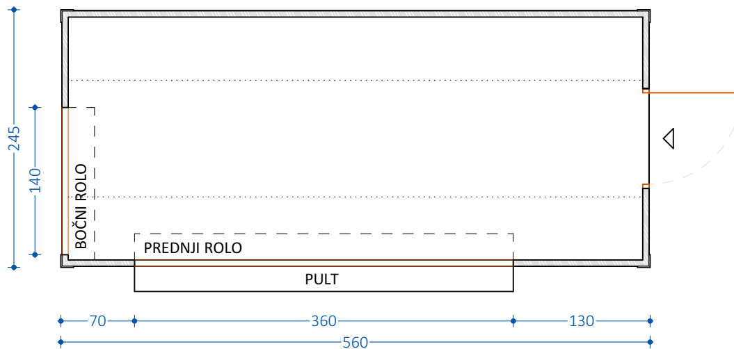
CAFFE BAR - TLOCRT
